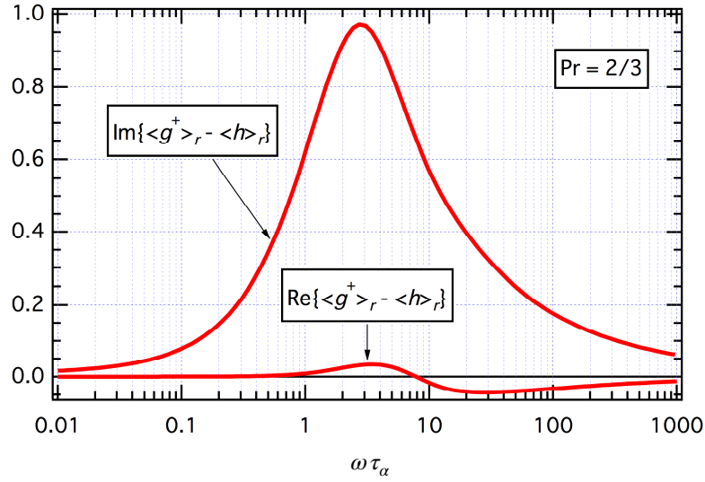
図13.1 プラントル数が2/3の場合の \langle g^\dagger \rangle_r - \langle h \rangle_r の \omega\tau_\alpha 依存性：実部は虚部に比べて著しく小さい。
