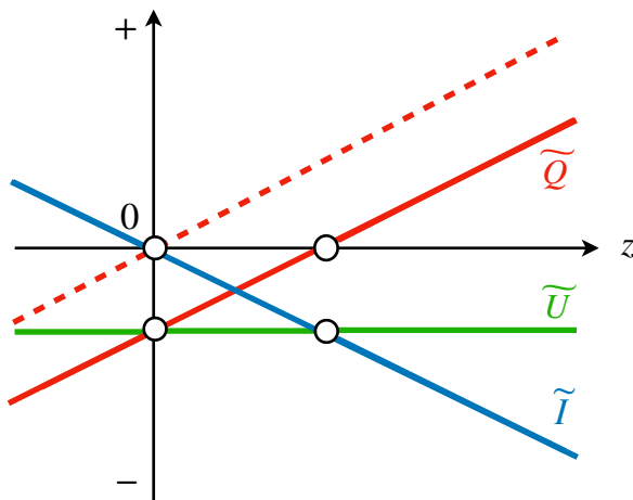
図12.2 強制振動 ( \nabla \tilde{Q} = -\nabla \tilde{I} > 0 ) の場合の仕事流密度 \tilde{I} 、熱流密度 \tilde{Q} 、エネルギー流密度 \tilde{U} \leq 0 の分布の模式図：熱音響ヒートポンプでは \tilde{Q} > 0 ですがドリームパイプでは \tilde{Q} < 0 です。破線は \tilde{U} = 0 の場合の熱流密度の分布です。
