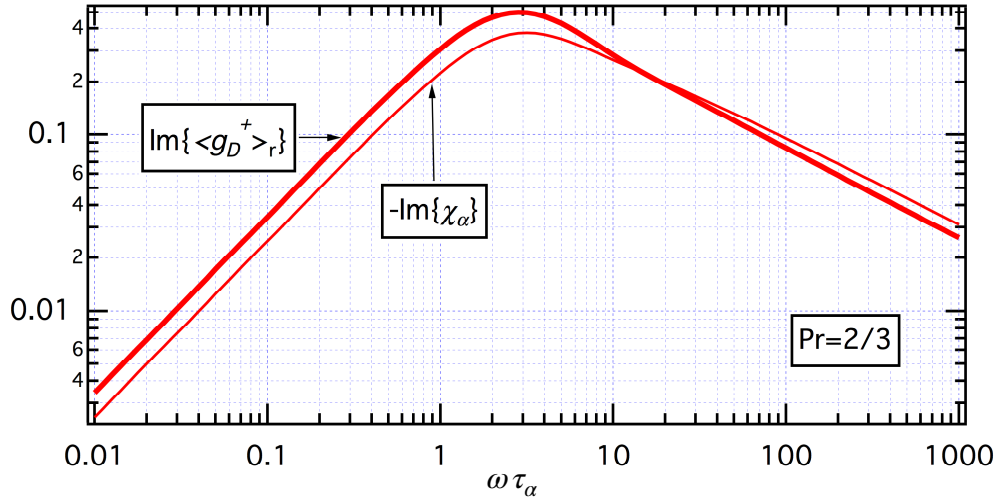
図12.3 \text{Pr} = 2/3 の場合の \Im\langle g_D^+ \rangle_r の \omega\tau_\alpha 依存性：比較のために \Im\chi_\alpha も示した。これは両対数グラフです。 \omega\tau_\alpha \leq \sqrt{10} では、 \Im\langle g_D^+ \rangle_r / \Im\chi_\alpha^\dagger \simeq 11/8 \simeq 1.4 です。
