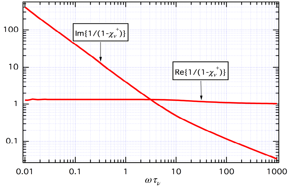
図11.2 1/(1 - \chi_\nu^\dagger) の \omega\tau_\nu 依存性：両対数表示です。 1/(1 - \chi_\nu^\dagger) の実数部は \omega\tau_\nu < 1 では 4/3 に近く、 \omega\tau_\nu > 10 では 1 に近い。 1/(1 - \chi_\nu^\dagger) の虚数部は \omega\tau_\nu の減少関数です。 \omega\tau_\nu < 1 では \omega\tau_\nu に反比例し、 \omega\tau_\nu > 10 では \sqrt{\omega\tau_\nu} に反比例している。
