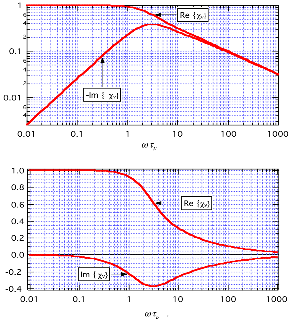
図8.1 \chi_\nu の \omega\tau_\nu 依存性：下図は片対数表示、上図は両対数表示です。上図のほうが漸近線の様子わかり易い。 \omega\tau_\nu \gg \sqrt{10} では粘性の影響が小さいが、 \omega\tau_\nu \ll \sqrt{10} では粘性の影響が大きい。
