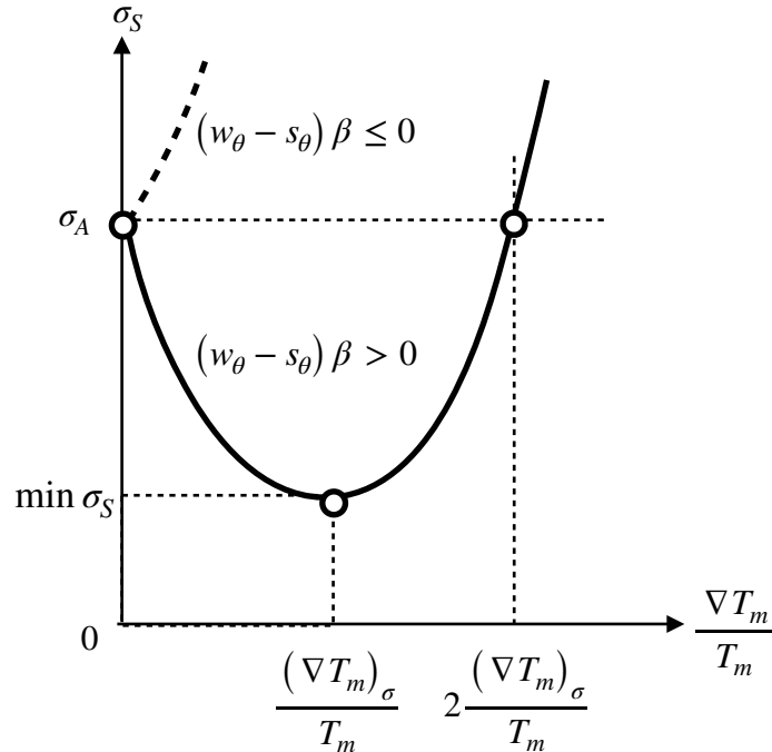
図12.5 熱音響理論のエントロピー生成密度 \sigma_S の \nabla T_m/T_m 依存性：破線は (w_\theta - s_\theta) \beta \leq 0 （破線）の場合には \sigma_S \geq \sigma_A です。 (w_\theta - s_\theta) \beta > 0 （実線）の場合には \nabla T_m/T_m = (\nabla T_m)_\sigma/T_m で最小値 \min \sigma_S < \sigma_A をとる。このためには \min \sigma_S \geq 0 も必要です。
