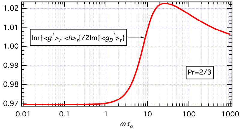
図13.2 プラントル数が2/3の場合の \Im(\langle g^\dagger \rangle_r - \langle h \rangle_r) / (2\Im\langle g_D^\dagger \rangle_r) の \omega\tau_\alpha 依存性： \Im(\langle g^\dagger \rangle_r - \langle h \rangle_r) と 2\Im\langle g_D^\dagger \rangle_r との相違は3%以下です。
