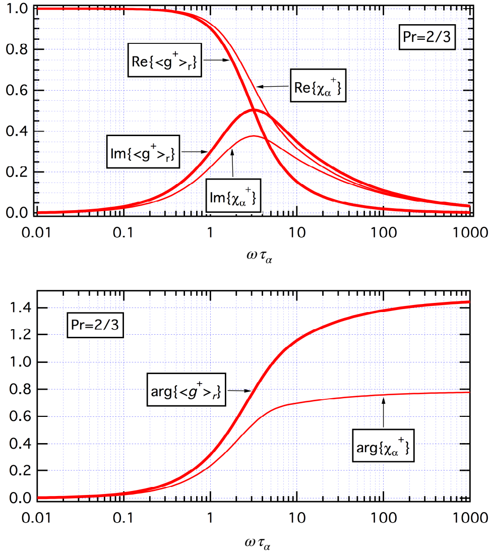
図12.4 Pr = 2/3 の場合の \langle g^+ \rangle_r の \omega\tau_\alpha 依存性：比較のために \chi_\alpha^+ も図示した。 \Re\langle g^+ \rangle_r < \Re\chi_\alpha^+ ですが、 \Im\langle g^+ \rangle_r > \Im\chi_\alpha^+ です。また、 0 < \arg\chi_\alpha^+ < \pi/4 ですが、 0 < \arg\langle g^+ \rangle_r < \pi/2 です。 \omega\tau_\alpha \simeq \pi で \arg\langle g^+ \rangle_r \simeq \pi/4 です。
