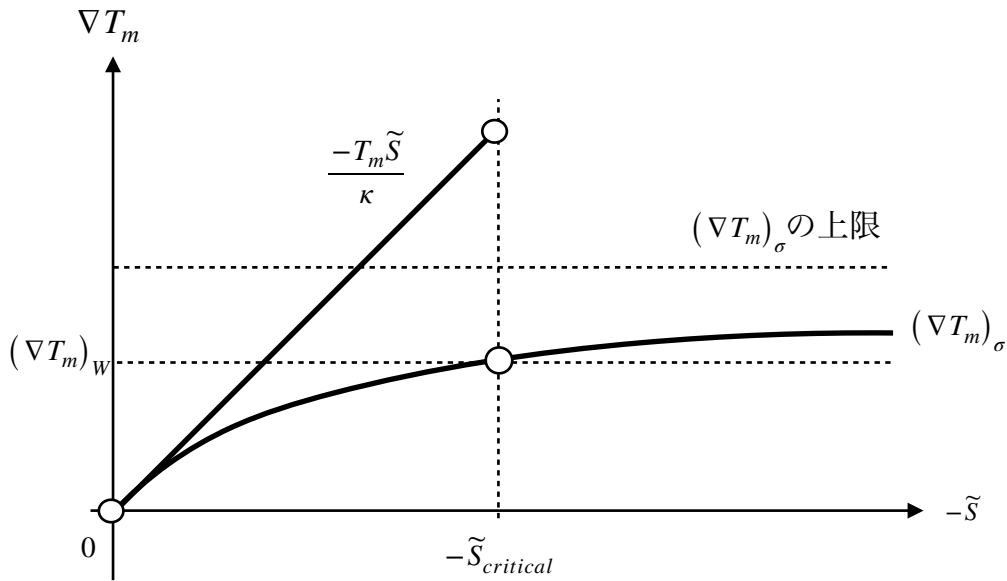
図13.3 単純熱伝導分岐 ( \nabla T_m = -T_m \tilde{S}/\kappa ) と熱音響自励振動分岐 ( \nabla T_m = (\nabla T_m)_\sigma ) の模式図： W > 0 となるのは、 \nabla T_m > (\nabla T_m)_W の領域だけです。 (\nabla T_m)_\sigma > (\nabla T_m)_W となるのは \tilde{S} > -\tilde{S}_{critical} の領域だけです。 0 < \tilde{S} < -\tilde{S}_{critical} では単純熱伝導分岐が安定に実現され、 \tilde{S} > -\tilde{S}_{critical} では熱音響自励振動分岐 (\nabla T_m)_\sigma が安定に実現される。高温部から低温部へ向かうエントロピー流の大きさ -\tilde{S} が大きくなって、 -\tilde{S} > -\tilde{S}_{critical} となると安定な熱音響自励振動が生じる。熱音響自励振動は散逸構造の一例です。
