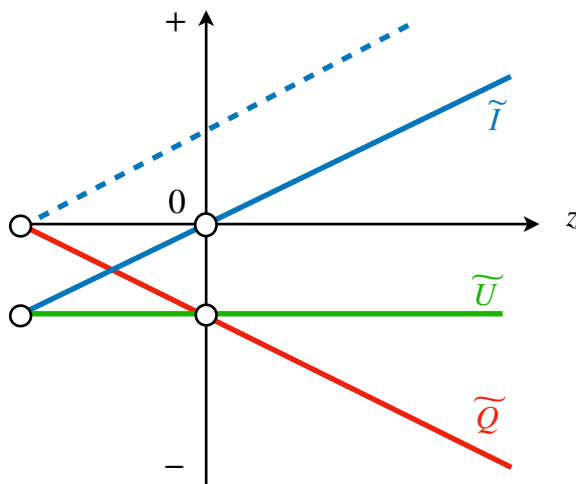
図12.1 自励振動 ( \nabla \tilde{I} = -\nabla \tilde{Q} > 0 ) の場合の仕事流密度 \tilde{I} 、熱流密度 \tilde{Q} < 0 、エネルギー流密度 \tilde{U} \leq 0 の分布の模式図： \tilde{I} < 0 の自励振動が可能なのは \tilde{U} < 0 の場合だけ。破線は \tilde{U} = 0 の場合の仕事流密度の分布です。
